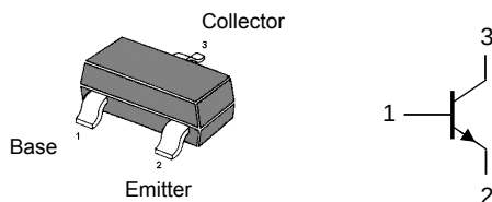
SOT-23
