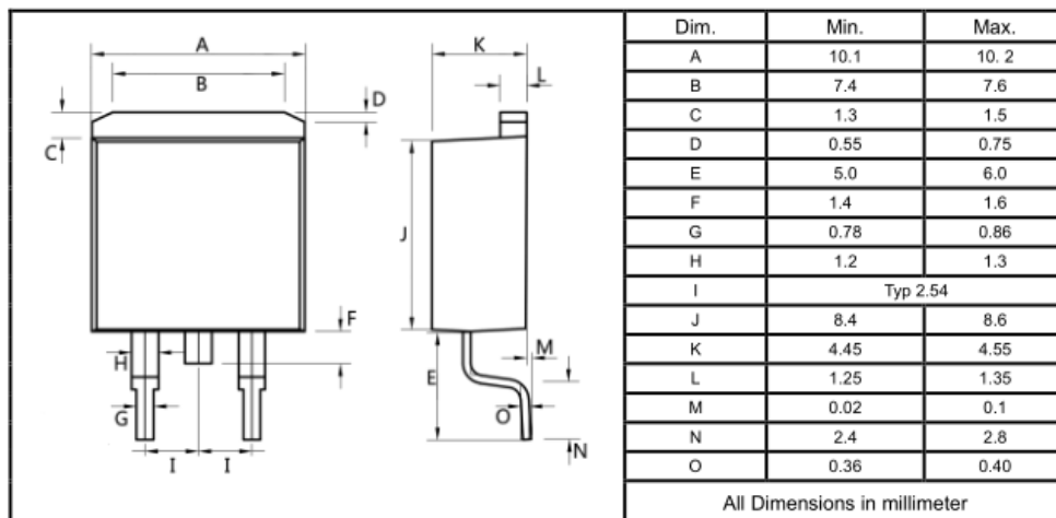
TO-263
