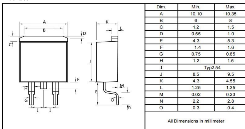
TO-263
