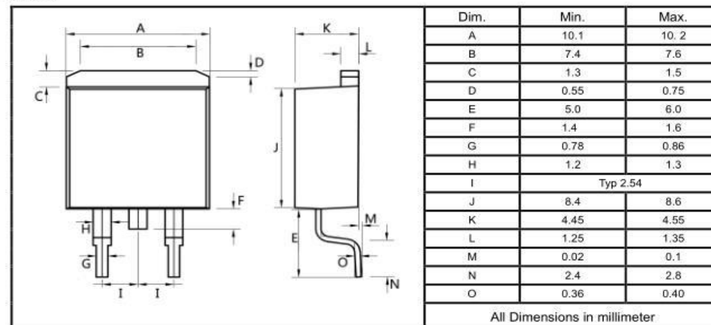
TO-263
