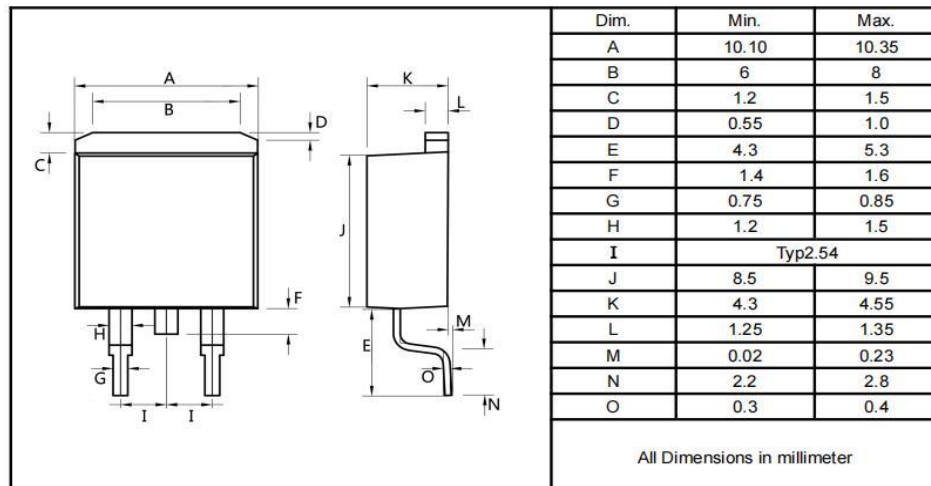
TO-263
